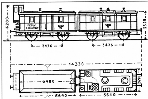
Železničný poštový vozň z roku 1858, názorné spojenie dvoch dvojnápravových vozňov do jedného štvornápravového vozňa
