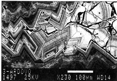
Obr.5 - Smithsonit v elektronovom mikroanalýzátore
